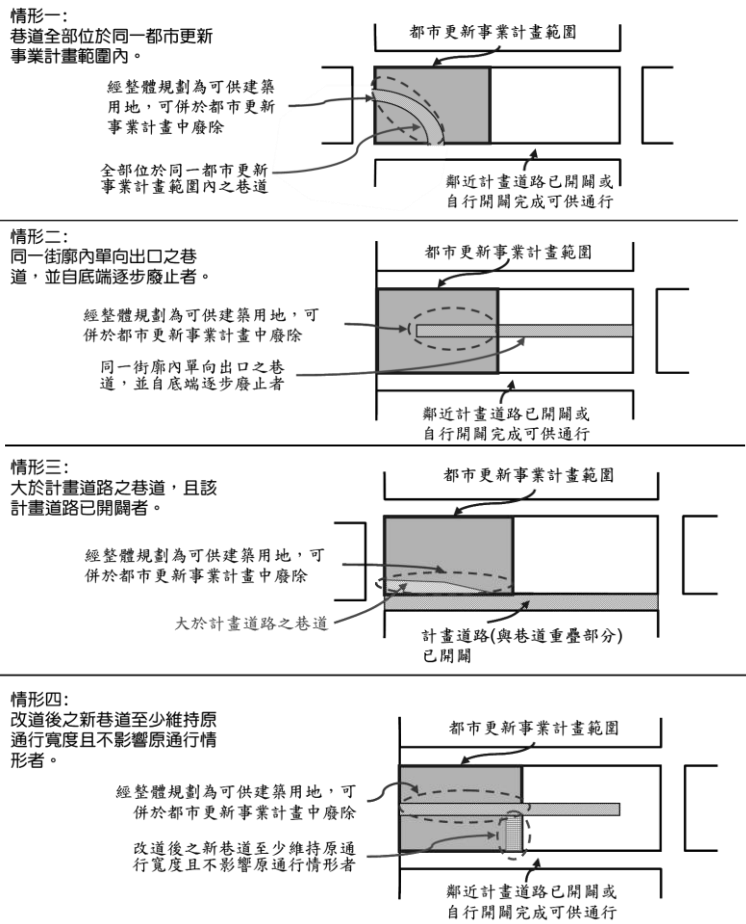
圖二：廢改道示意圖
