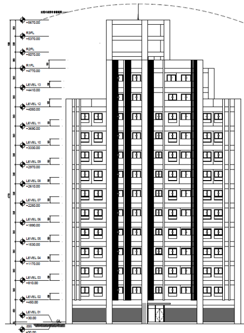
重建後建築立面圖
