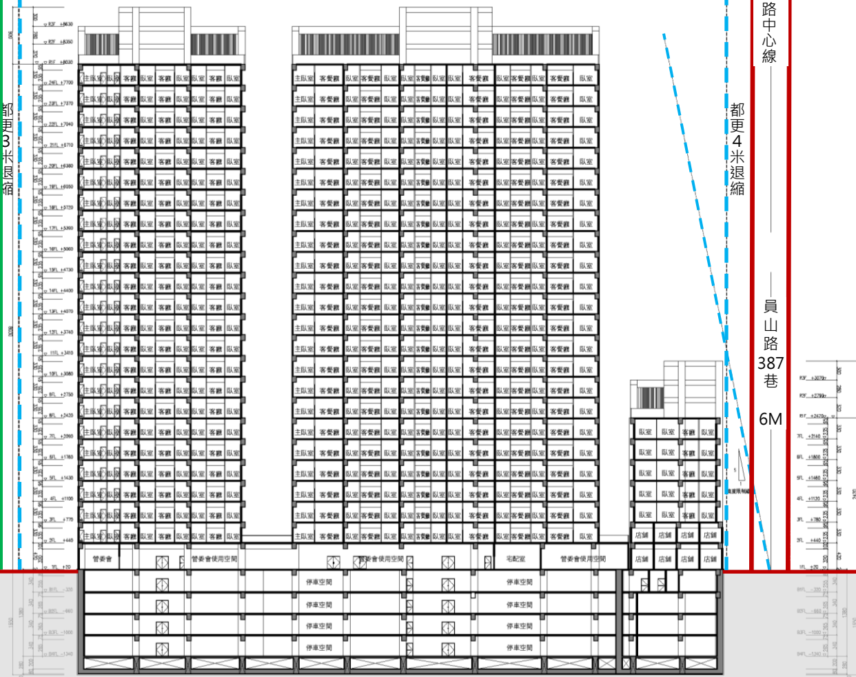
橫向剖面圖
