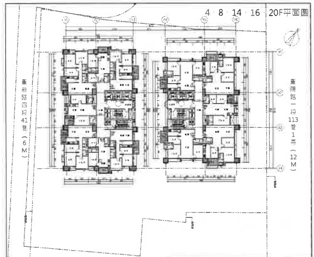
標準層平面圖
