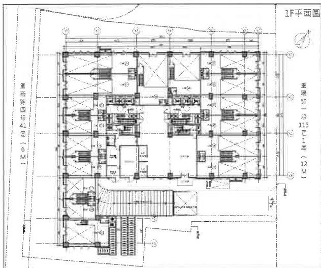
一樓平面圖
