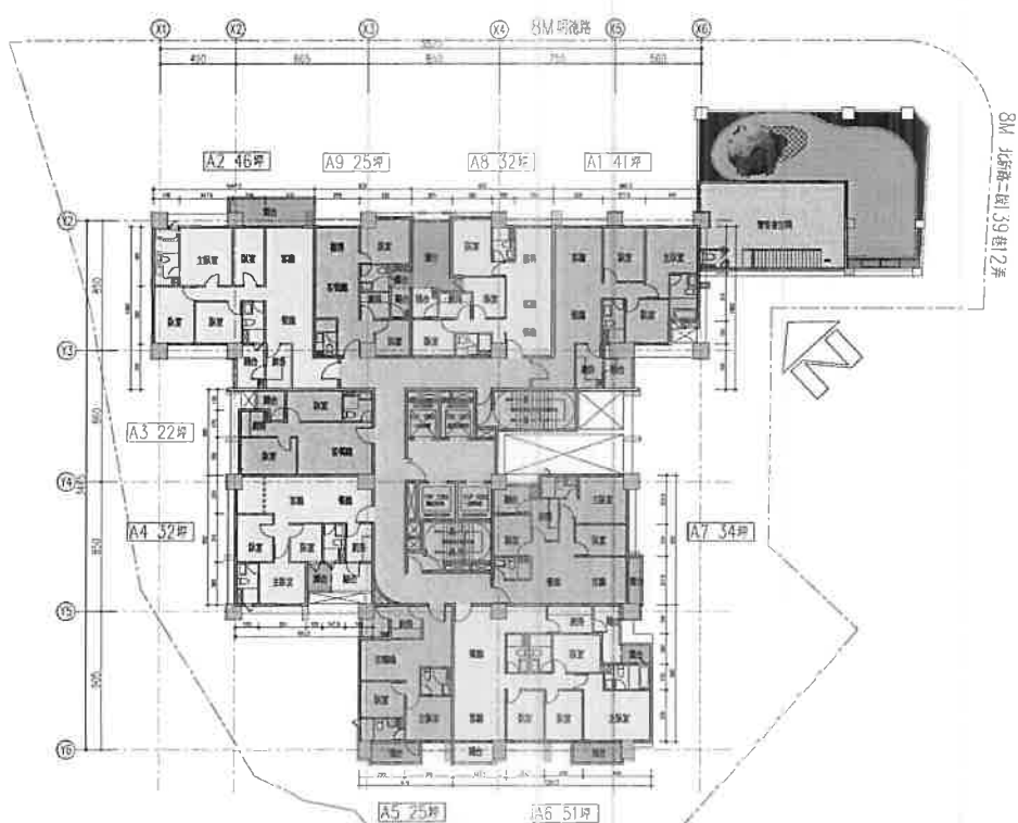
地上三層平面圖
