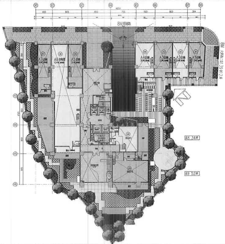
地上一層平面圖
