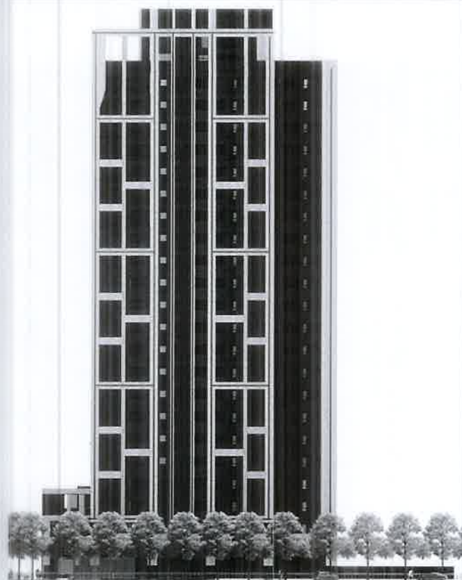
右向立面
